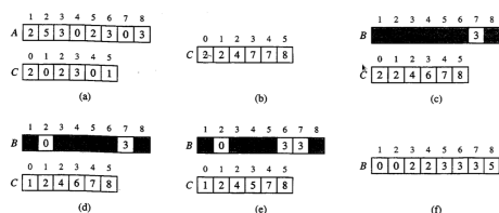
FIGURA 8.2 A operação de COUNTING-SORT sobre um arranjo de entrada A[1..8] , onde cada elemento de A é um inteiro não negativo não maior que k = 5 . (a) O arranjo A e o arranjo auxiliar C após a linha 4. (b) O arranjo C após a linha 7. (c)–(e) O arranjo de saída B e o arranjo auxiliar C após uma, duas e três iterações do loop nas linhas 9 a 11, respectivamente. Apenas os elementos levemente sombreados do arranjo B foram preenchidos. (f) O arranjo de saída final ordenado B
