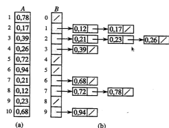
FIGURA 8.4 A operação de BUCKET-SORT. (a) O arranjo de entrada A[1..10] . (b) O arranjo B[0..9] de listas ordenadas (baldes) depois da linha 5 do algoritmo. O balde i contém valores no intervalo [i/10, (i+1)/10) . A saída ordenada consiste em uma concatenação em ordem das listas B[0], B[1], \dots, B[9]
